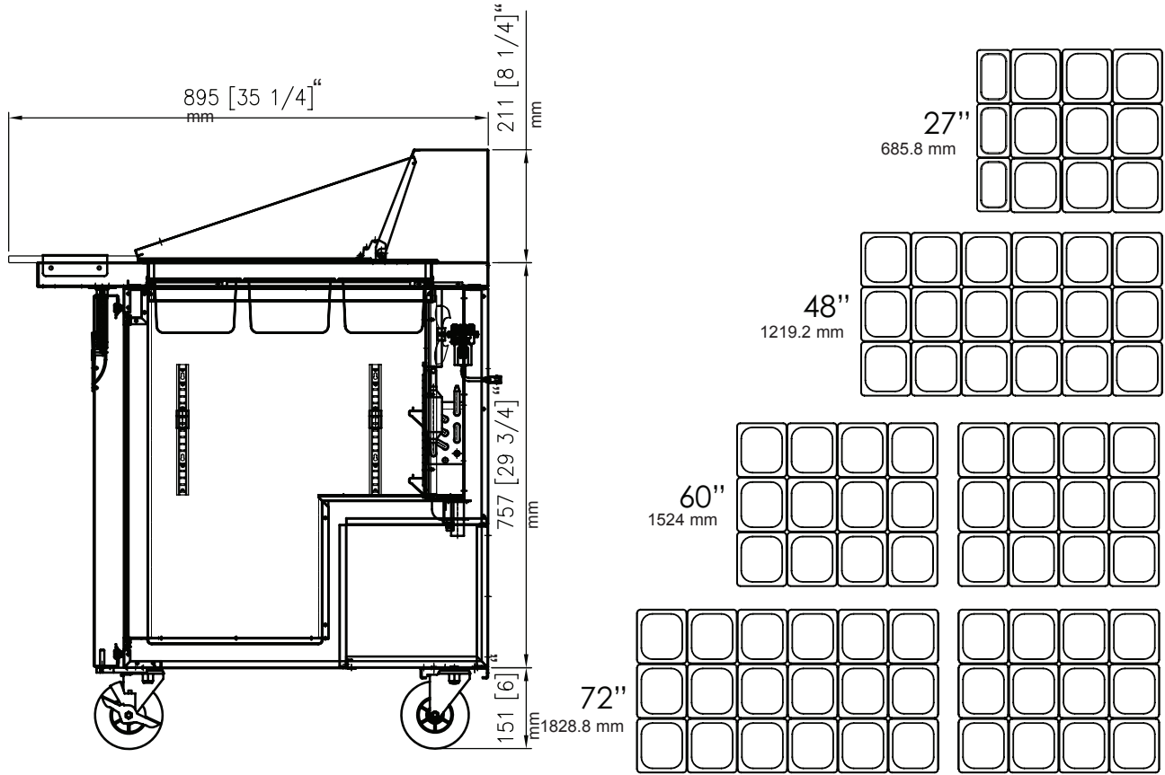
Megatop Pan Array
